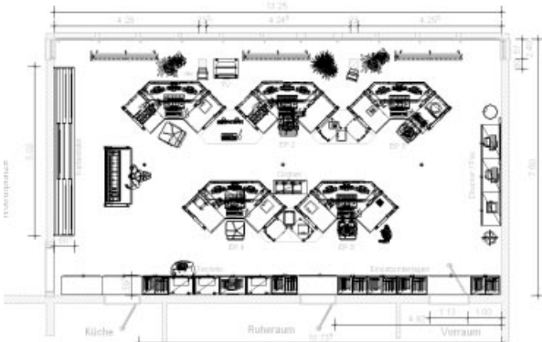
Grundrissplanung entsprechend arbeitstechnischer Abläufe und Platzbedarf
